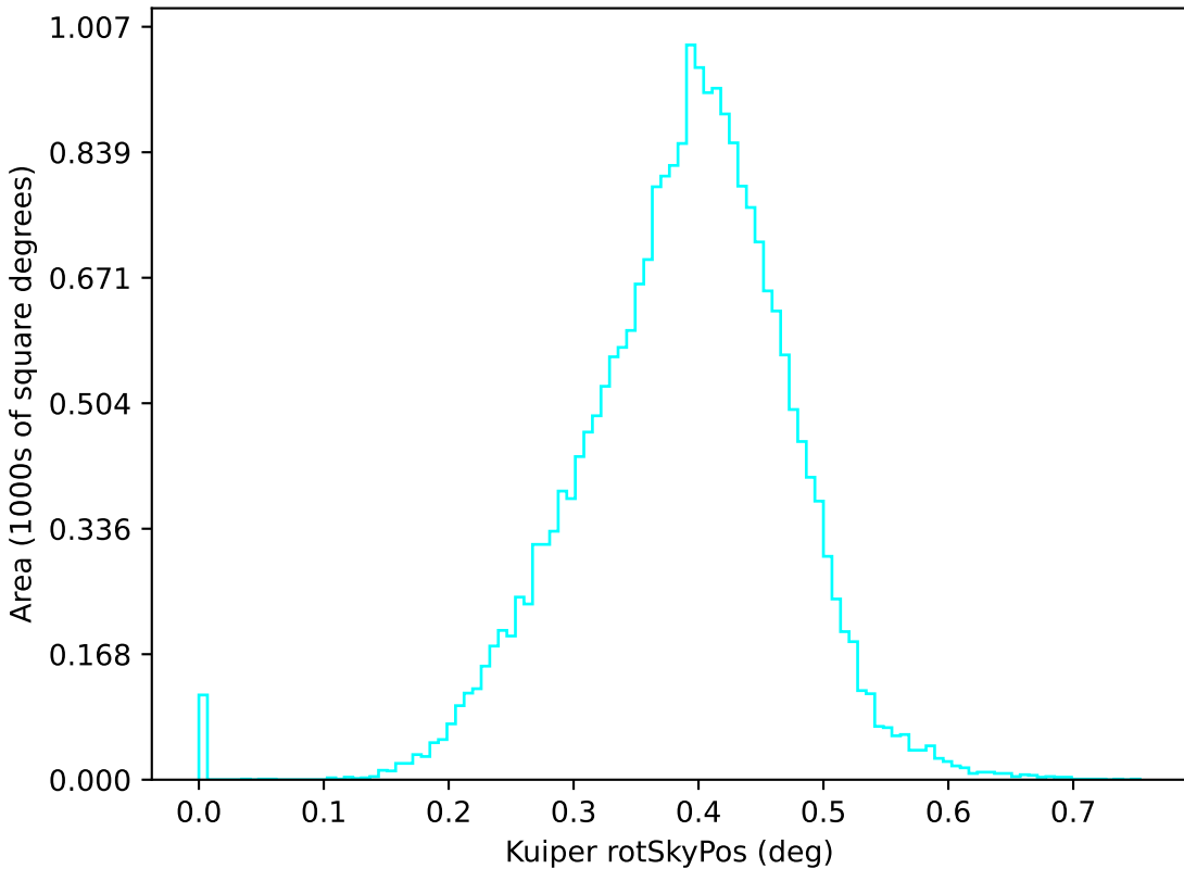
all_long_v3.4_10yrs u: Kuiper rotSkyPos
