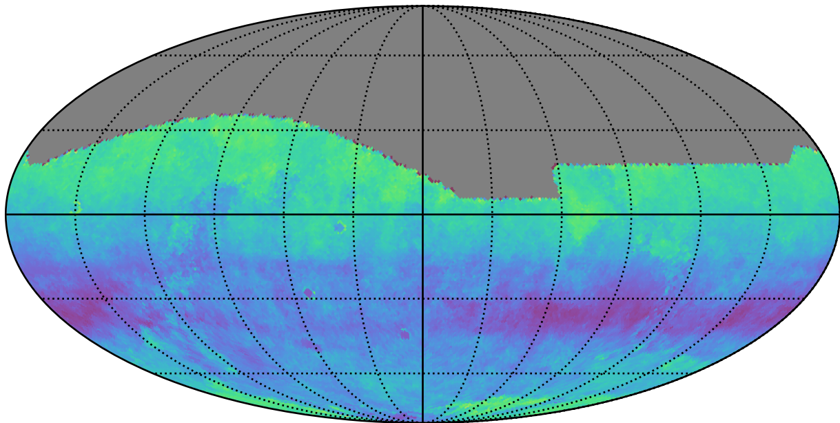
all_long_v3.4_10yrs r: Kuiper rotSkyPos
