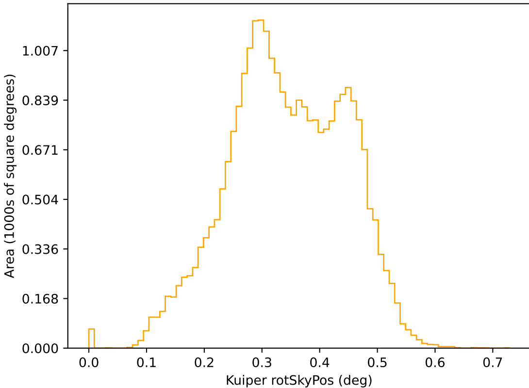
all_long_v3.4_10yrs r: Kuiper rotSkyPos
