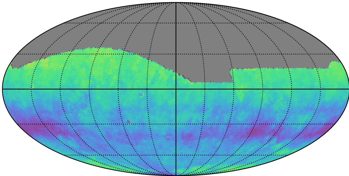
all_long_v3.4_10yrs i: Kuiper rotSkyPos
