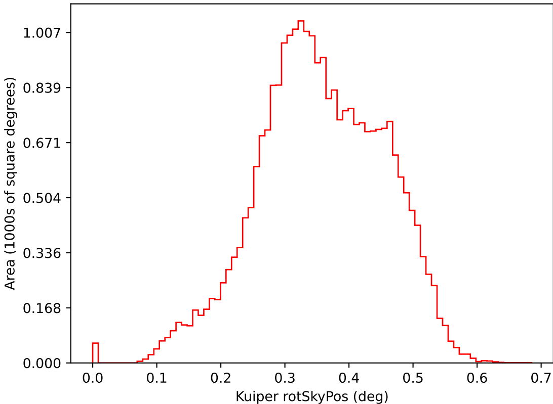
all_long_v3.4_10yrs i: Kuiper rotSkyPos
