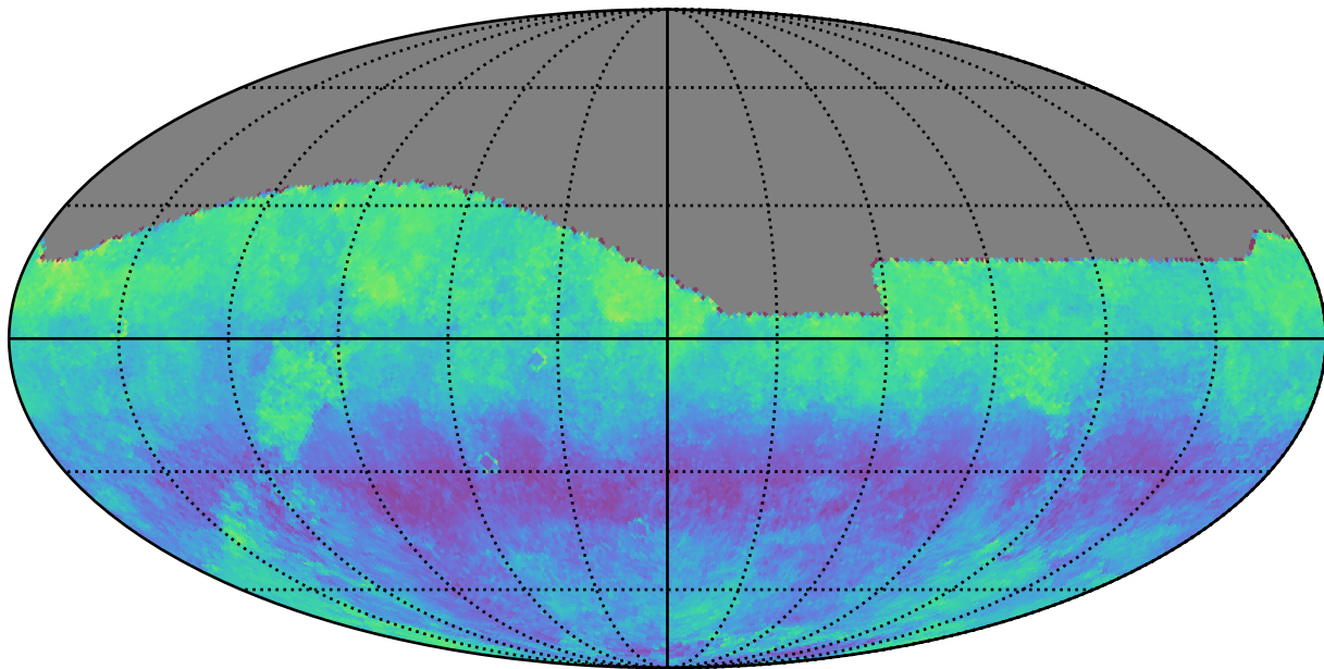
all_long_v3.4_10yrs g: Kuiper rotSkyPos
