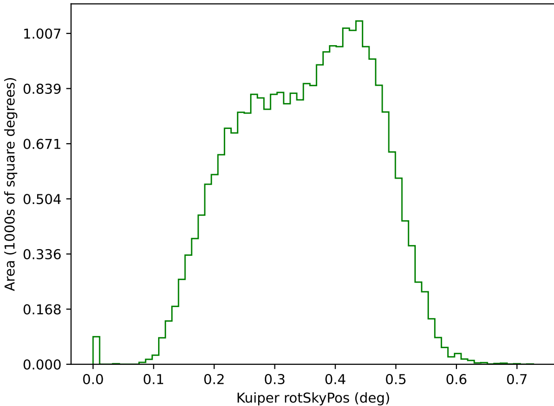
all_long_v3.4_10yrs g: Kuiper rotSkyPos
