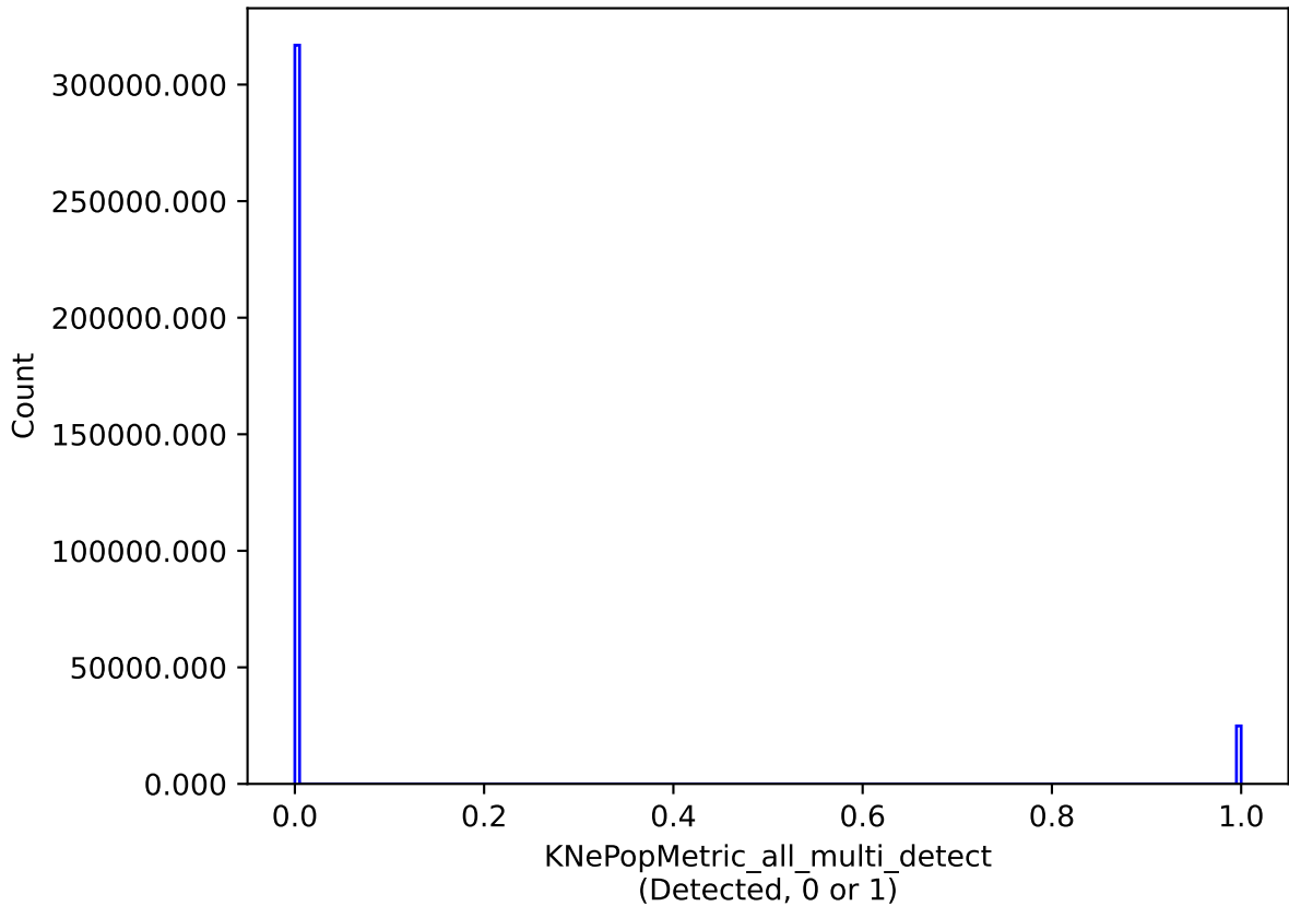
all_long_v3.4_10yrs all models: KNePopMetric_all_multi_detect
