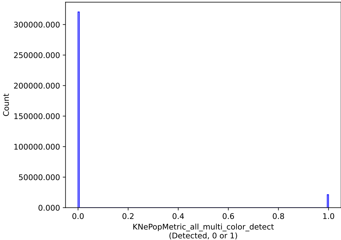
all_long_v3.4_10yrs all models: KNePopMetric_all_multi_color_detect
