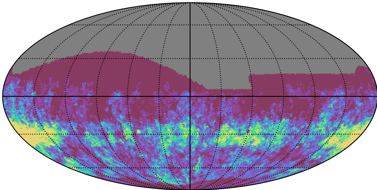
all_long_v3.4_10yrs i band: Gaps_7hr
