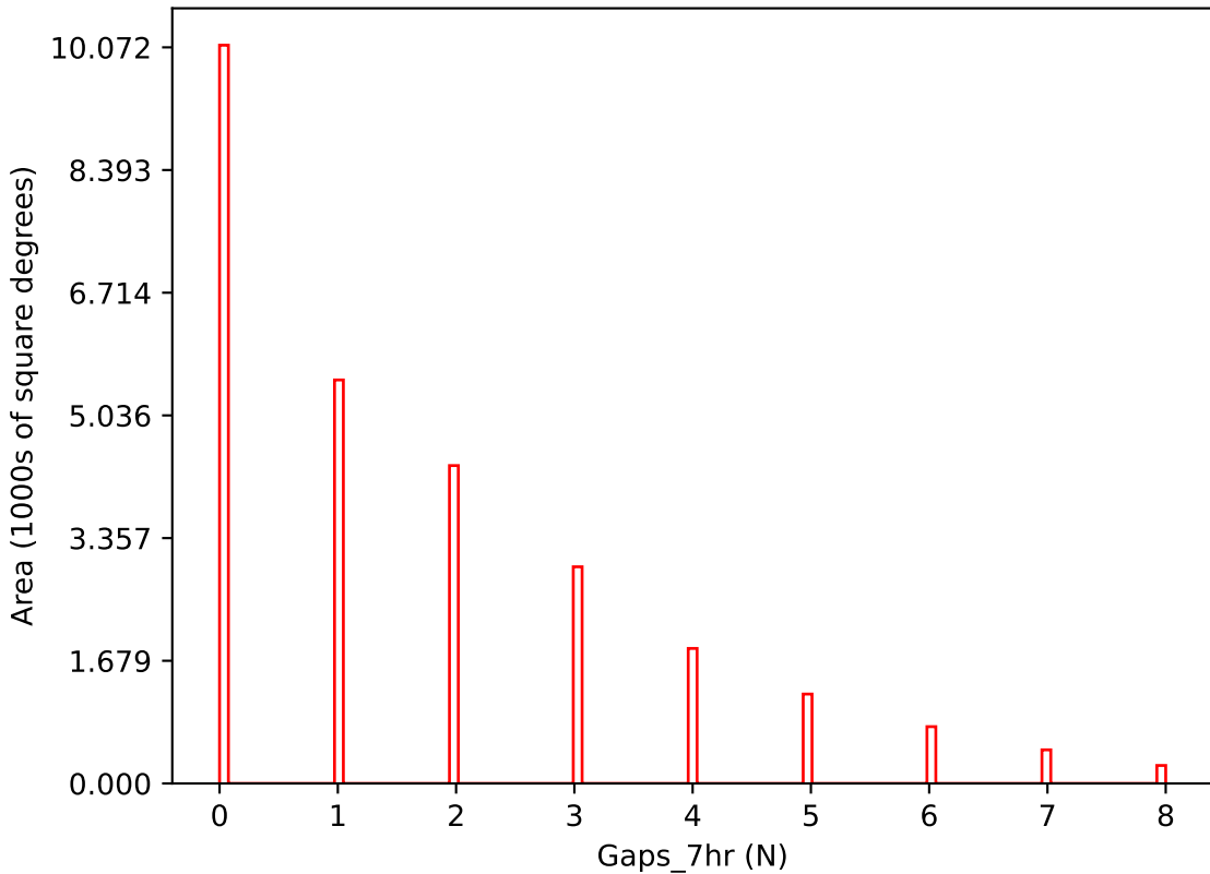
all_long_v3.4_10yrs i band: Gaps_7hr
