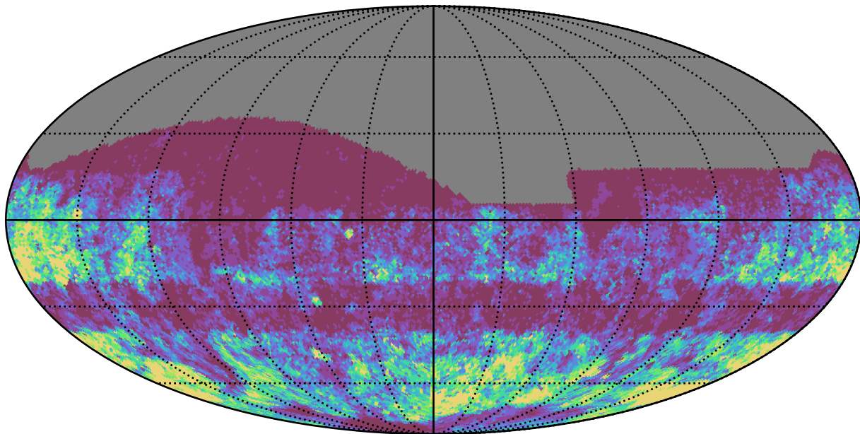
all_long_v3.4_10yrs i band: Gaps_3hr
