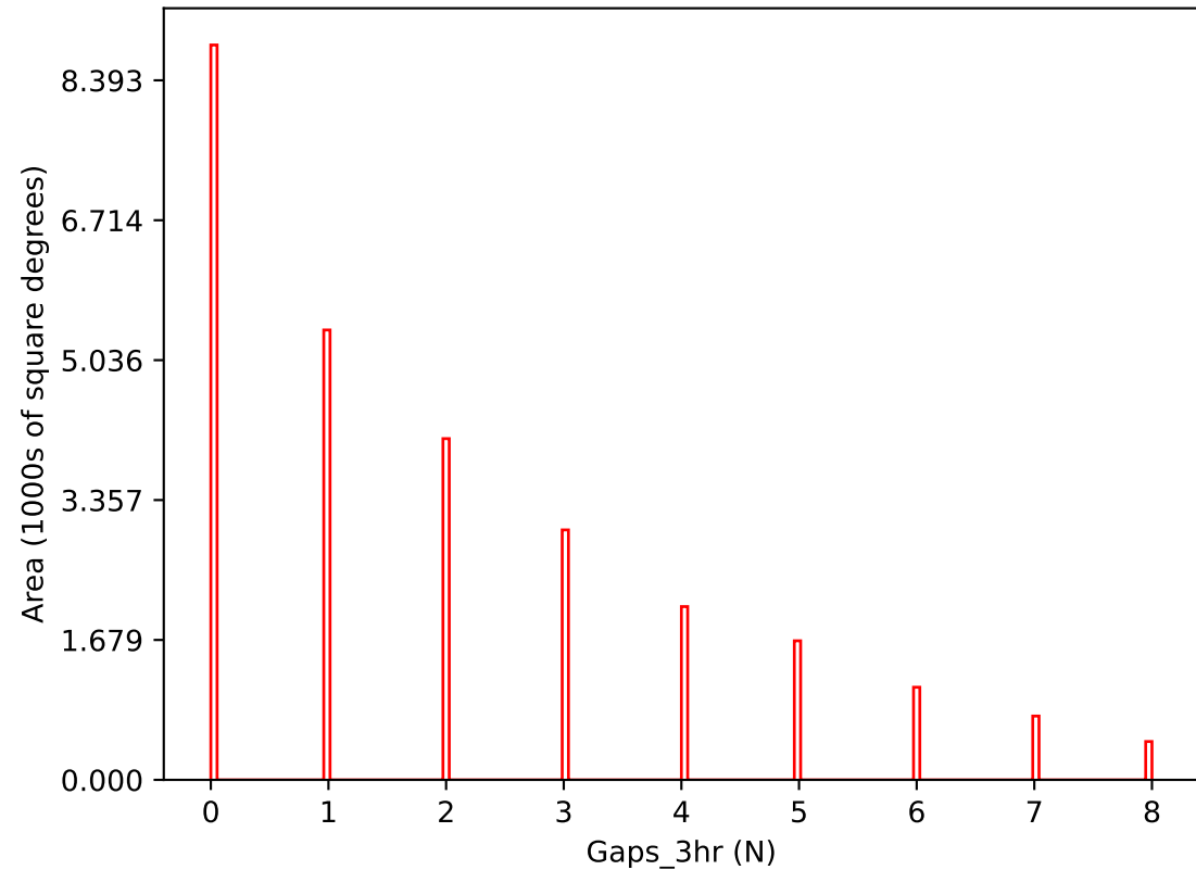
all_long_v3.4_10yrs i band: Gaps_3hr
