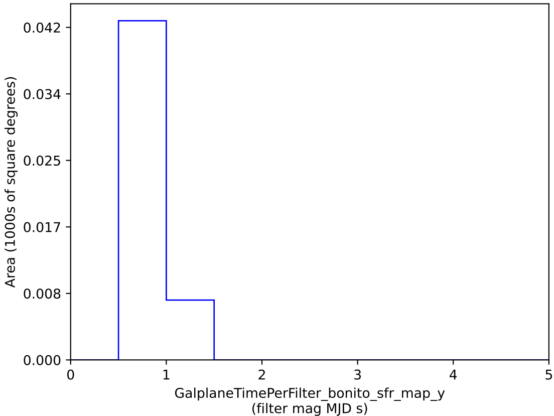
all_long_v3.4_10yrs : GalplaneTimePerFilter_bonito_sfr_map_y
