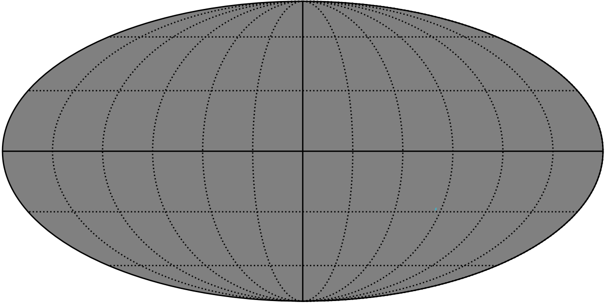
all_long_v3.4_10yrs : GalplaneFootprintMetric_globular_clusters_map_Tau_46_5
