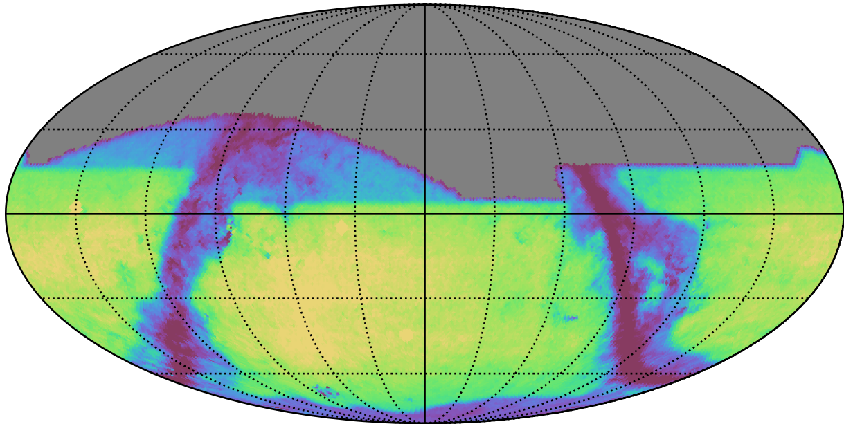
all_long_v3.4_10yrs i: GalaxyCountsMetricExtended
