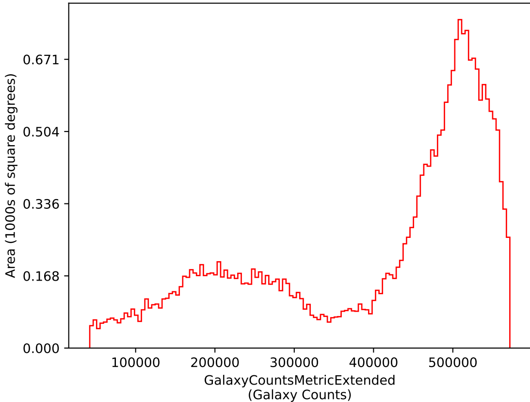
all_long_v3.4_10yrs i: GalaxyCountsMetricExtended
