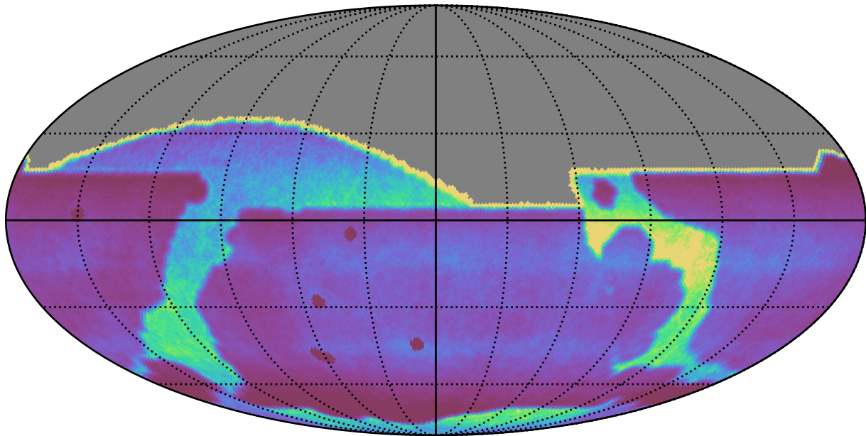
all_long_v3.4_10yrs : DCRprecision
