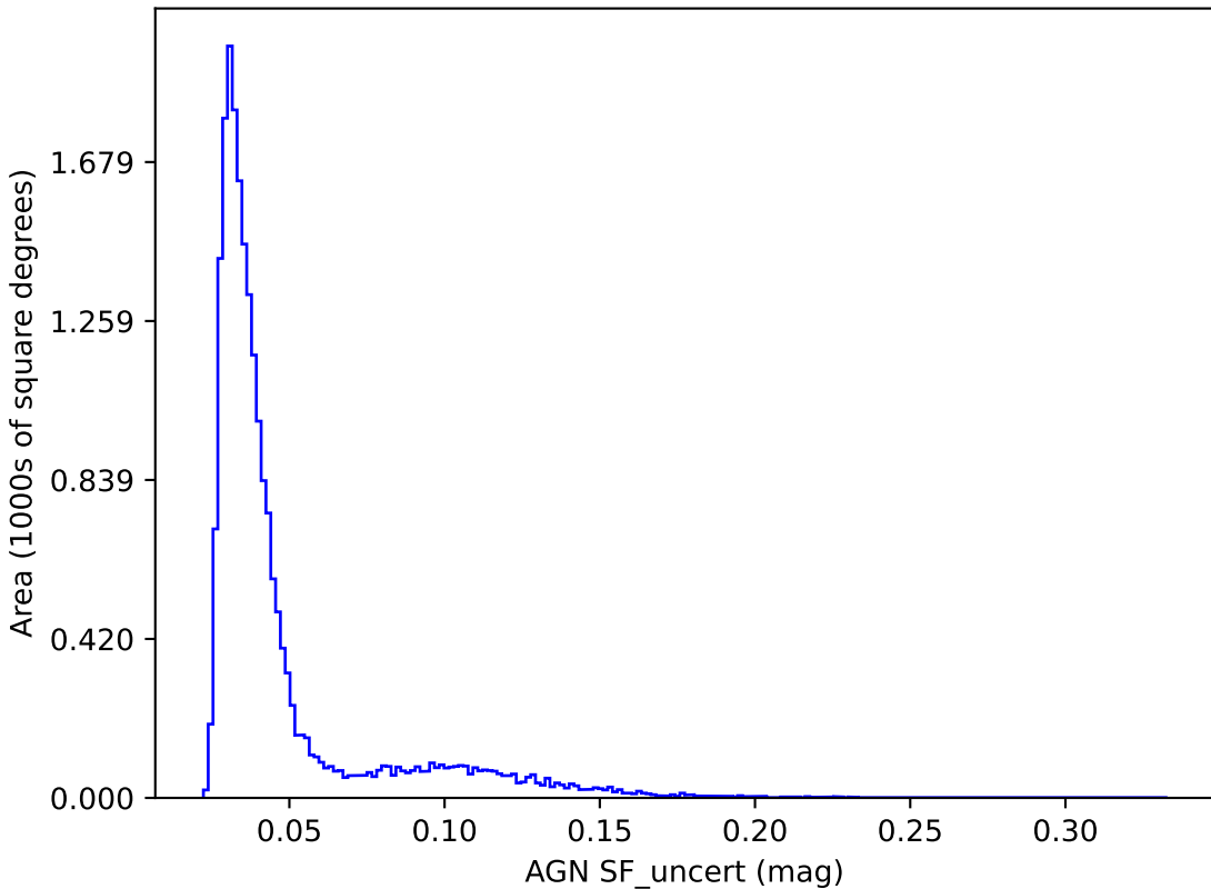
all_long_v3.4_10yrs y band: AGN SF_uncert
