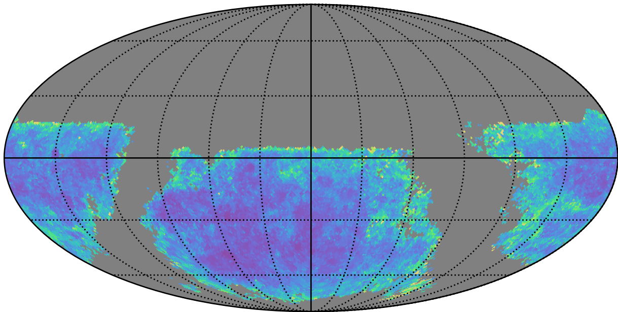
all_long_v3.4_10yrs u band: AGN SF_uncert
