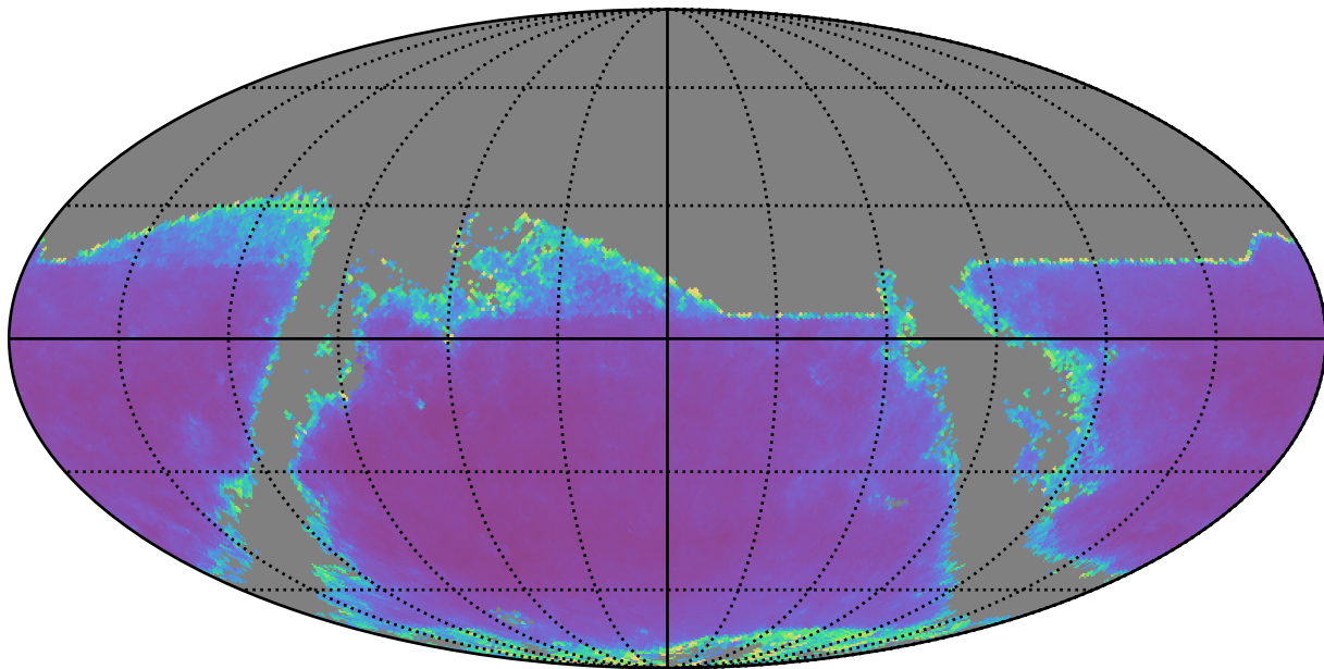
all_long_v3.4_10yrs r band: AGN SF_uncert
