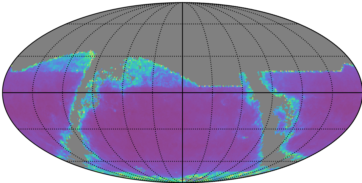
all_long_v3.4_10yrs i band: AGN SF_uncert
