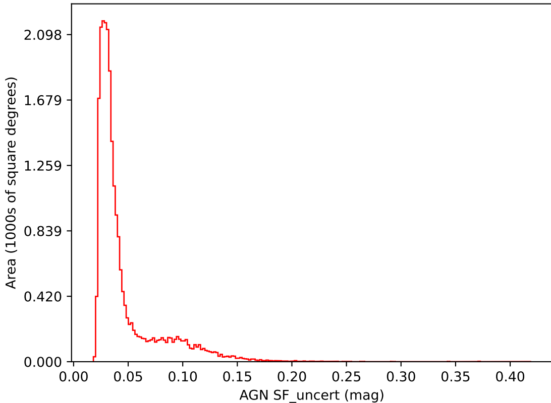
all_long_v3.4_10yrs i band: AGN SF_uncert
