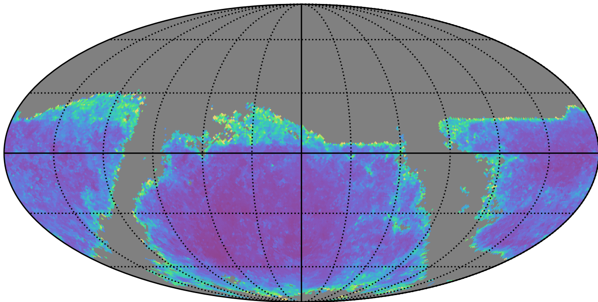
all_long_v3.4_10yrs g band: AGN SF_uncert
