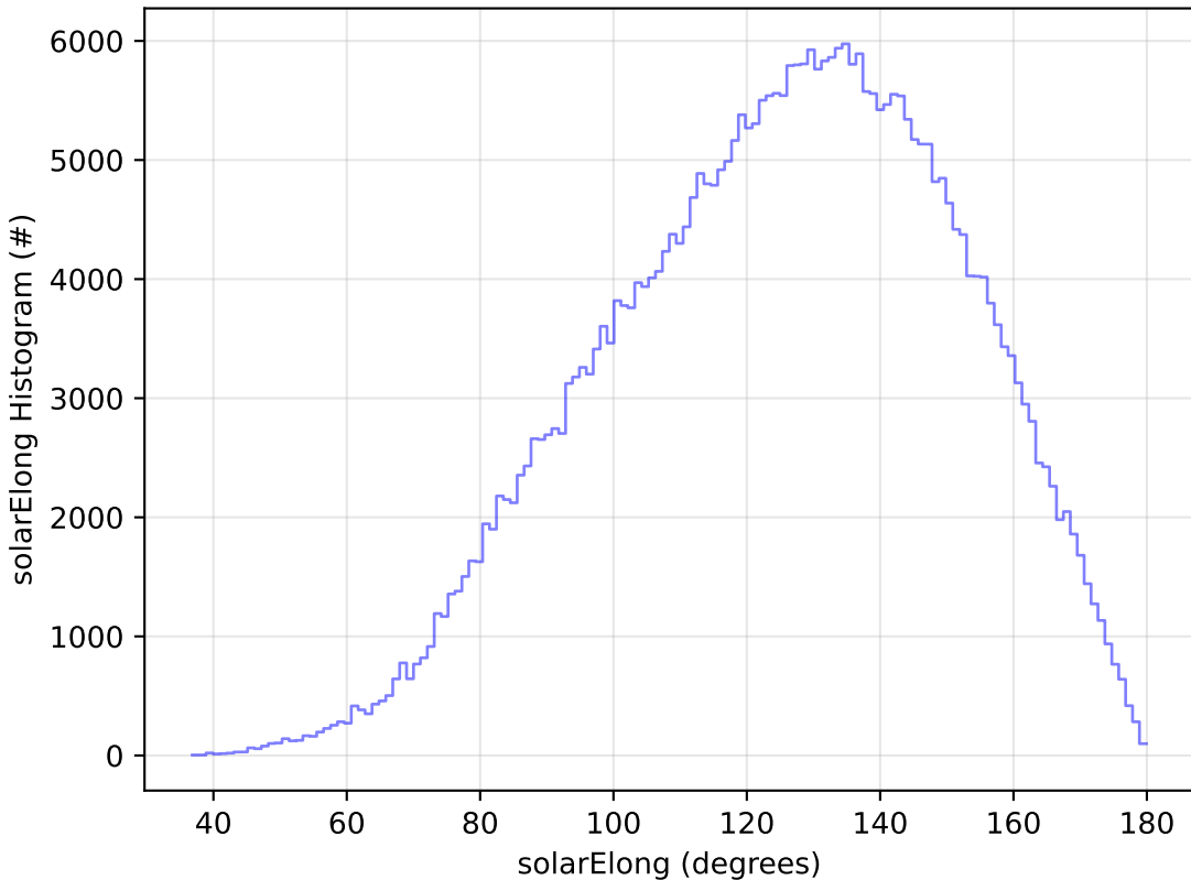
all_long_v3.4_10yrs All sky y band: solarElong Histogram
