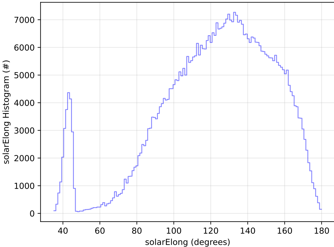
all_long_v3.4_10yrs All sky i band: solarElong Histogram
