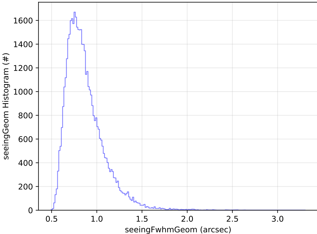
all_long_v3.4_10yrs Yr 1 y band: seeingGeom Histogram
