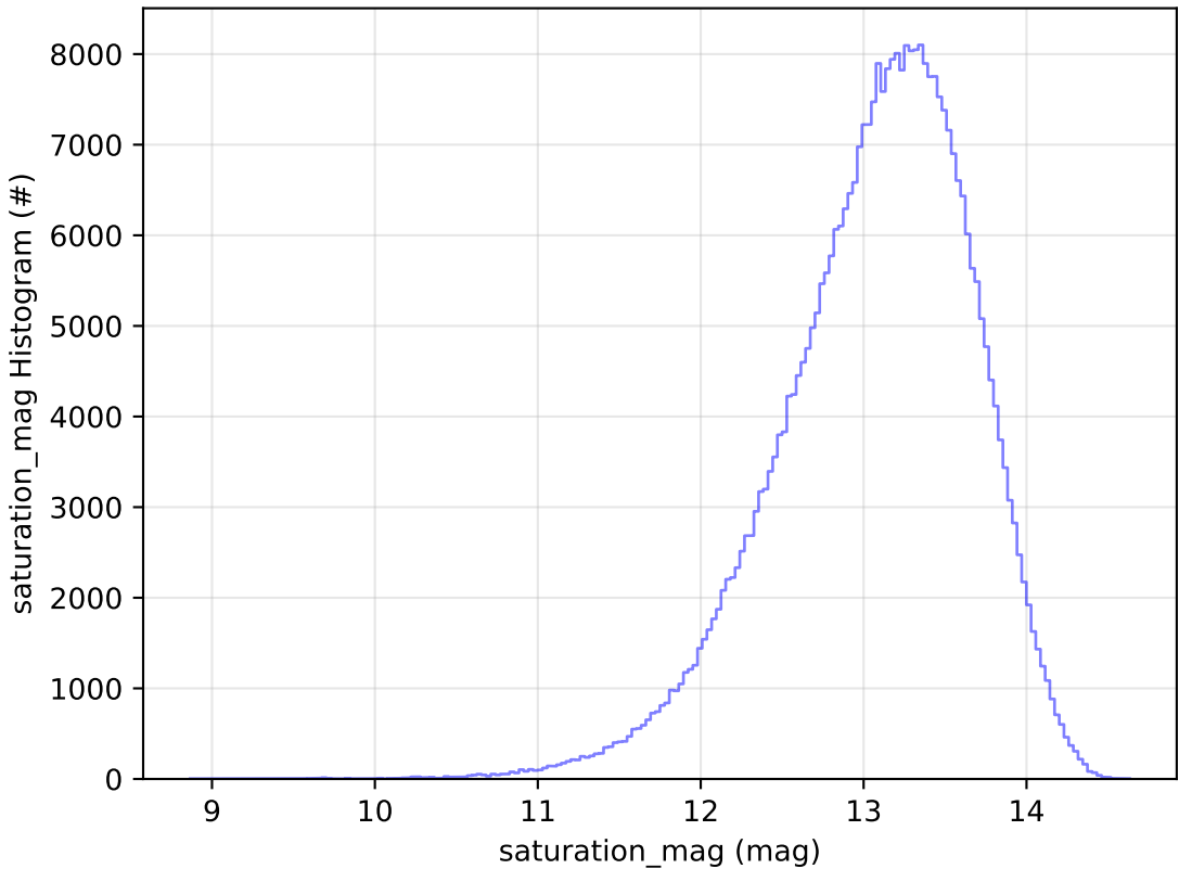
all_long_v3.4_10yrs WFD y band: saturation_mag Histogram
