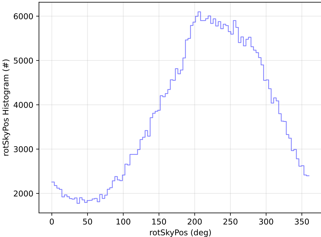
all_long_v3.4_10yrs WFD y band: rotSkyPos Histogram
