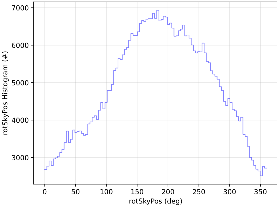
all_long_v3.4_10yrs All sky i band: rotSkyPos Histogram
