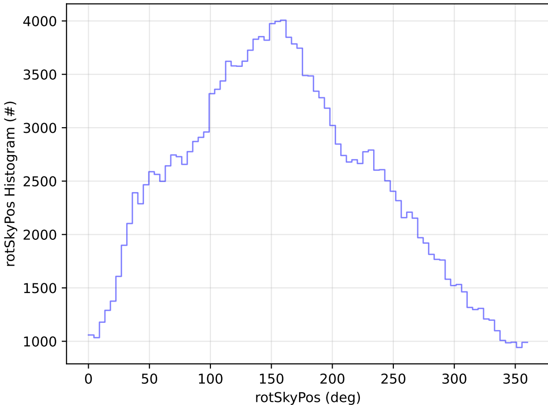
all_long_v3.4_10yrs All sky g band: rotSkyPos Histogram
