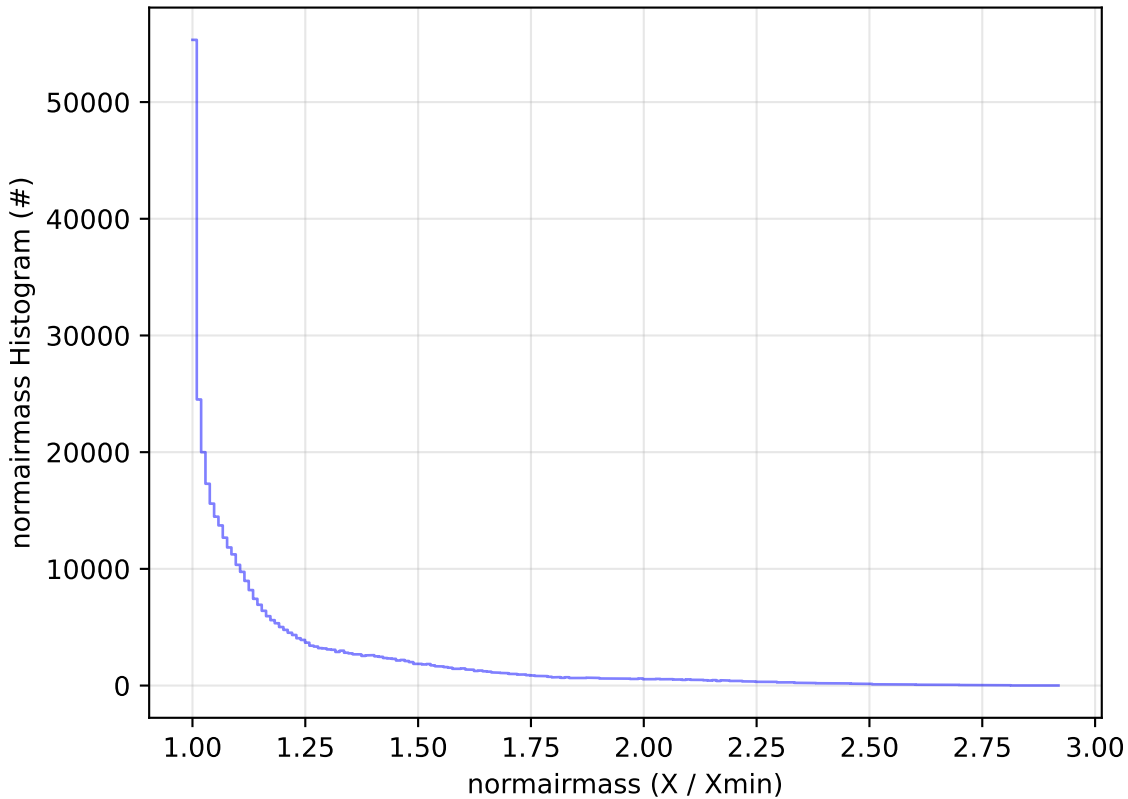
all_long_v3.4_10yrs WFD z band: normairmass Histogram
