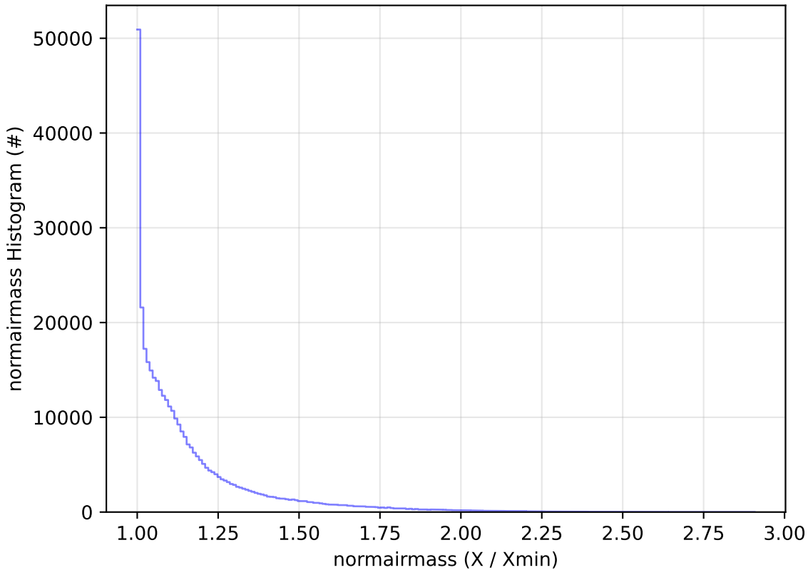
all_long_v3.4_10yrs All sky y band: normairmass Histogram
