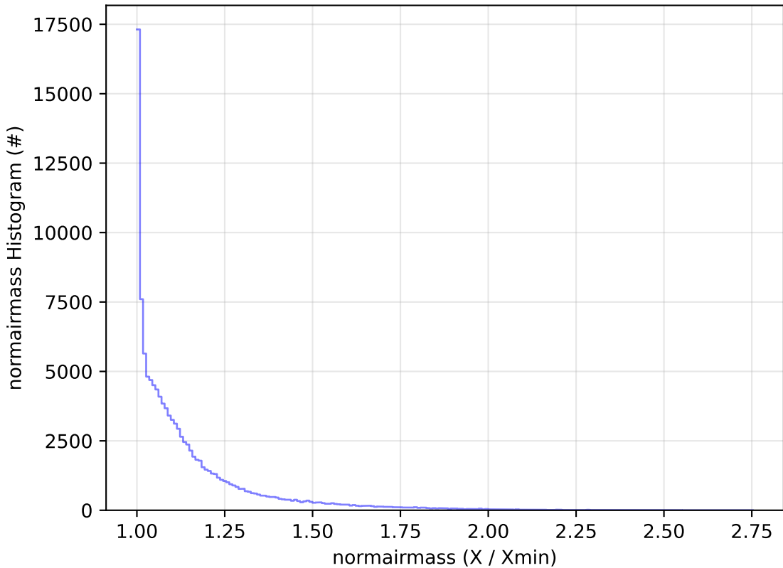
all_long_v3.4_10yrs All sky u band: normairmass Histogram
