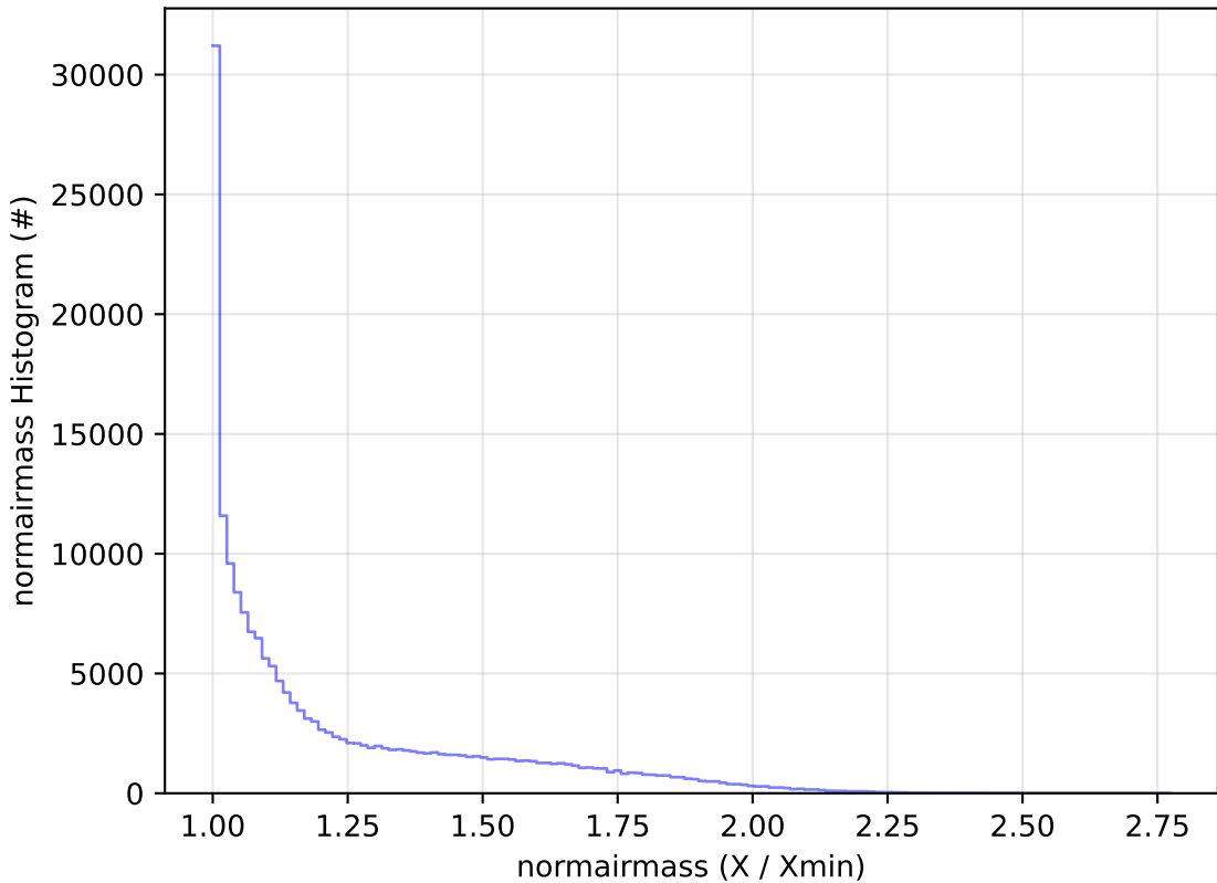
all_long_v3.4_10yrs All sky g band: normairmass Histogram
