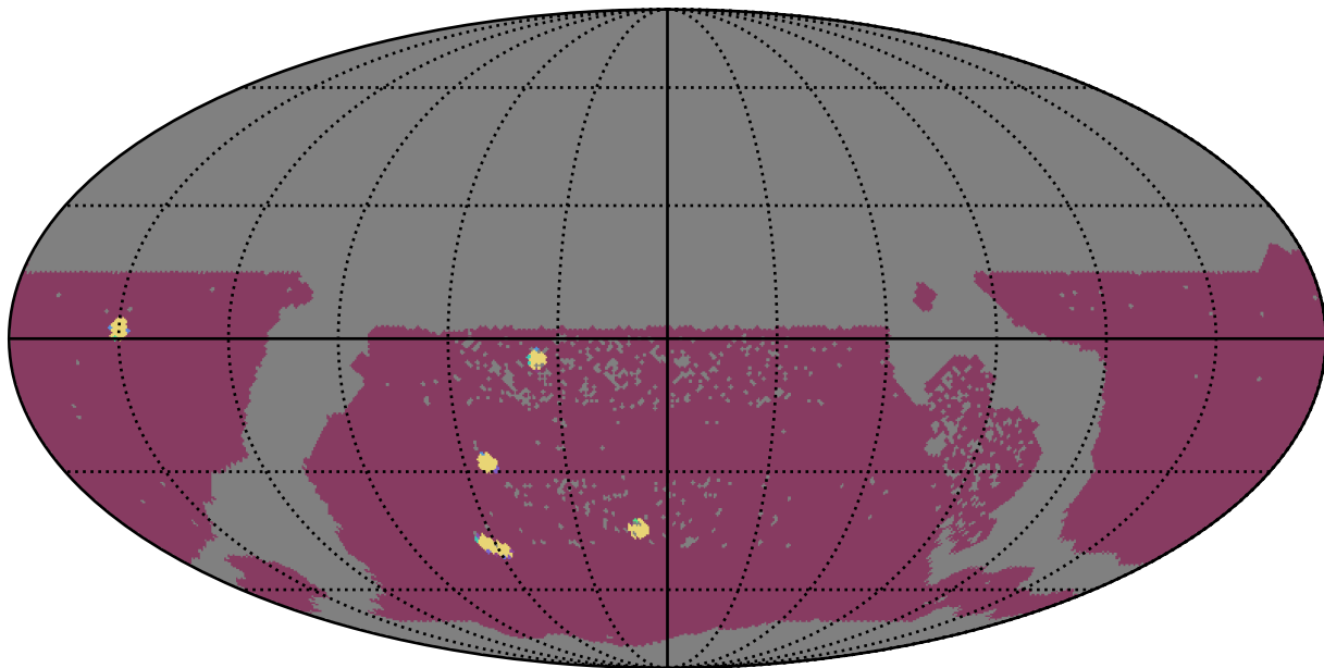
all_long_v3.4_10yrs WFD: NumberOfQuickRevisits
