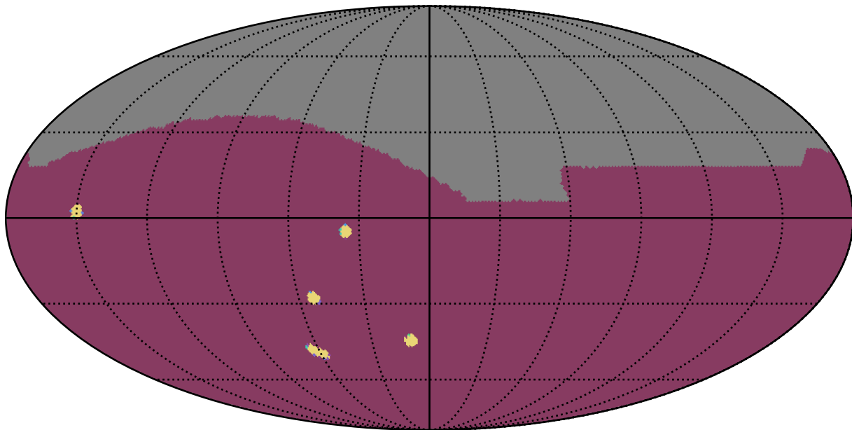
all_long_v3.4_10yrs All sky: NumberOfQuickRevisits
