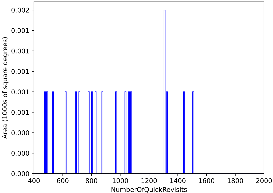
all_long_v3.4_10yrs All sky: NumberOfQuickRevisits
