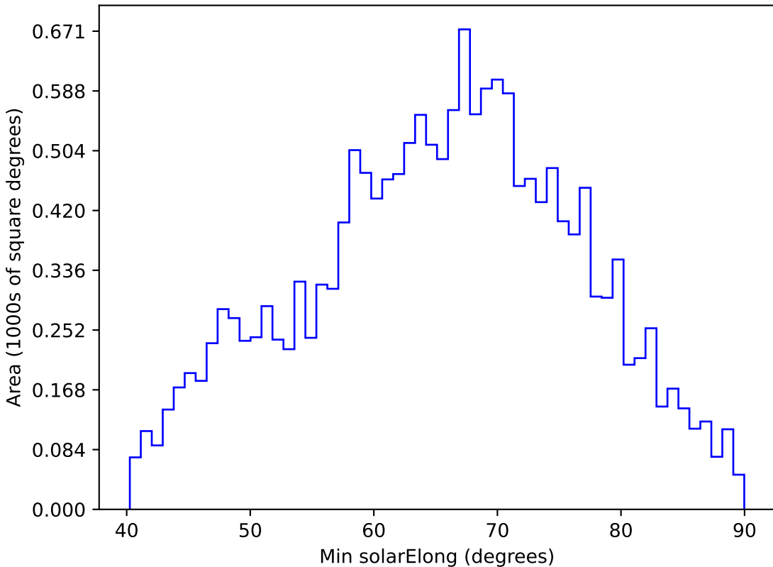
all_long_v3.4_10yrs WFD y band: Min solarElong
