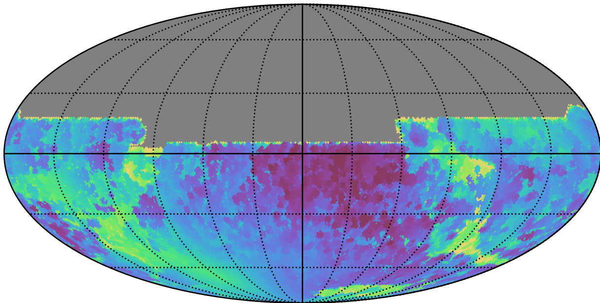
all_long_v3.4_10yrs All sky y band: Min solarElong
