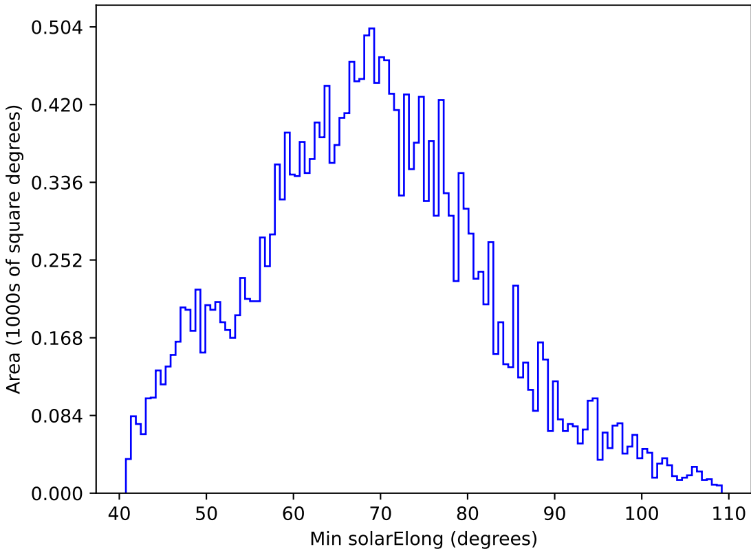
all_long_v3.4_10yrs All sky y band: Min solarElong
