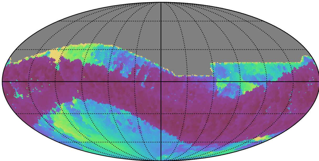
all_long_v3.4_10yrs All sky i band: Min solarElong
