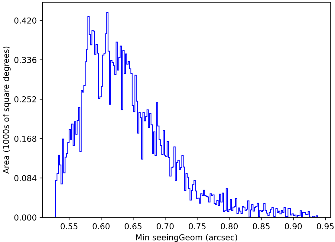
all_long_v3.4_10yrs Yr 1 y band: Min seeingGeom
