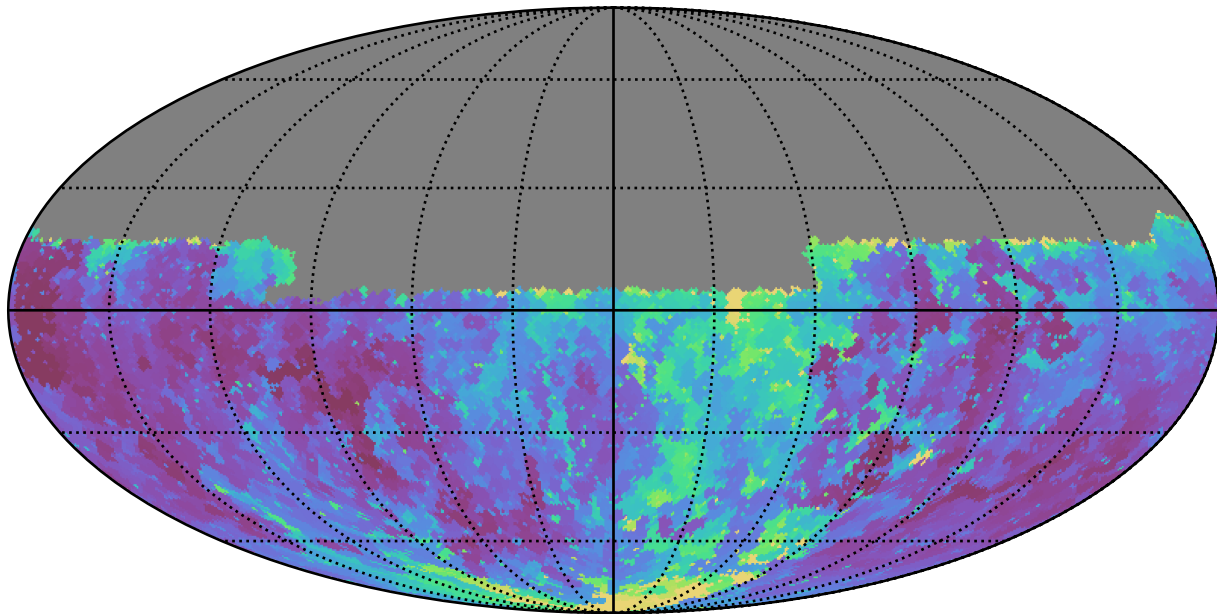
all_long_v3.4_10yrs Yr 1 u band: Min seeingGeom
