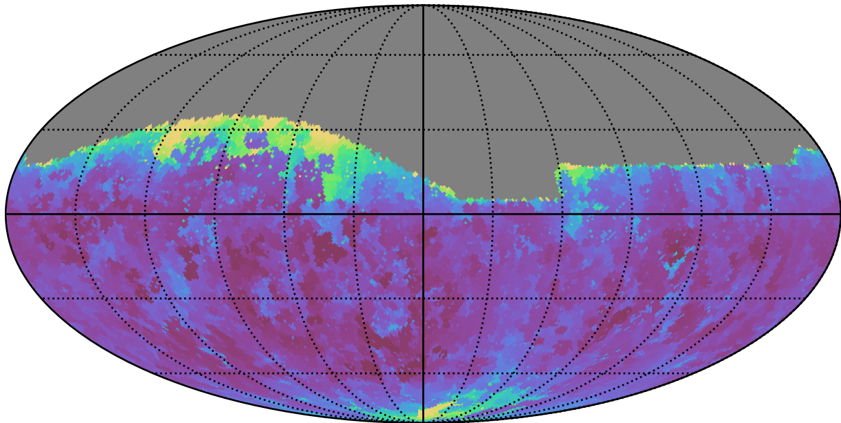
all_long_v3.4_10yrs Yr 1 r band: Min seeingGeom
