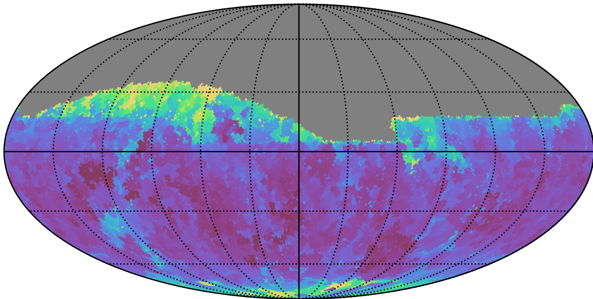
all_long_v3.4_10yrs Yr 1 i band: Min seeingGeom
