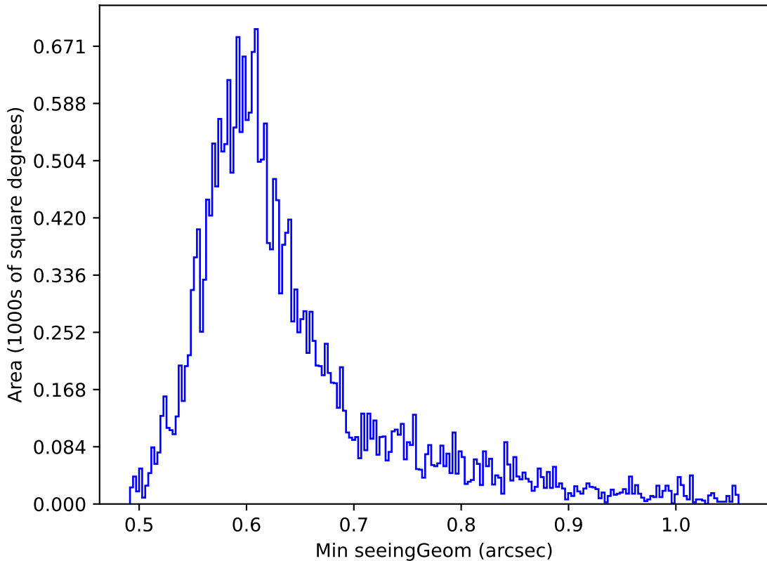
all_long_v3.4_10yrs Yr 1 i band: Min seeingGeom
