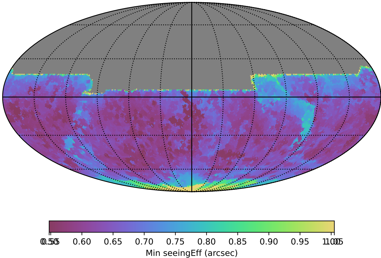
all_long_v3.4_10yrs All sky y band: Min seeingEff
