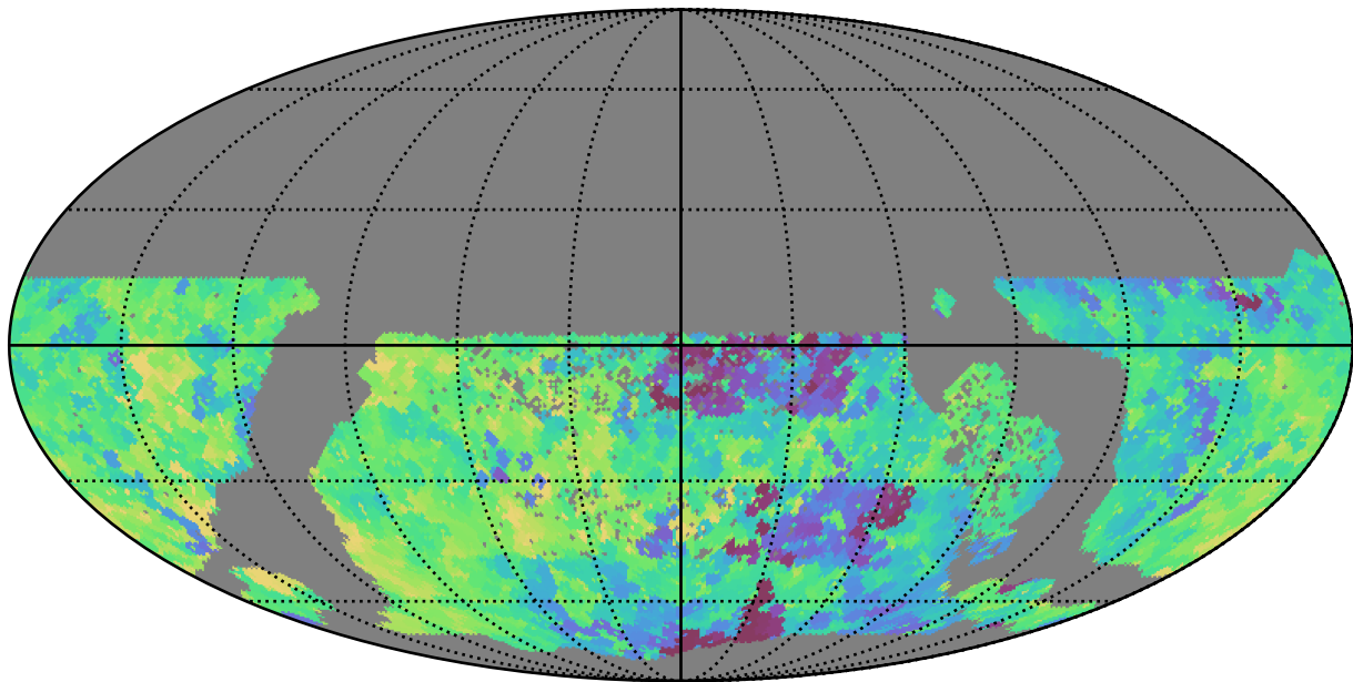
all_long_v3.4_10yrs WFD y band: Min saturation_mag
