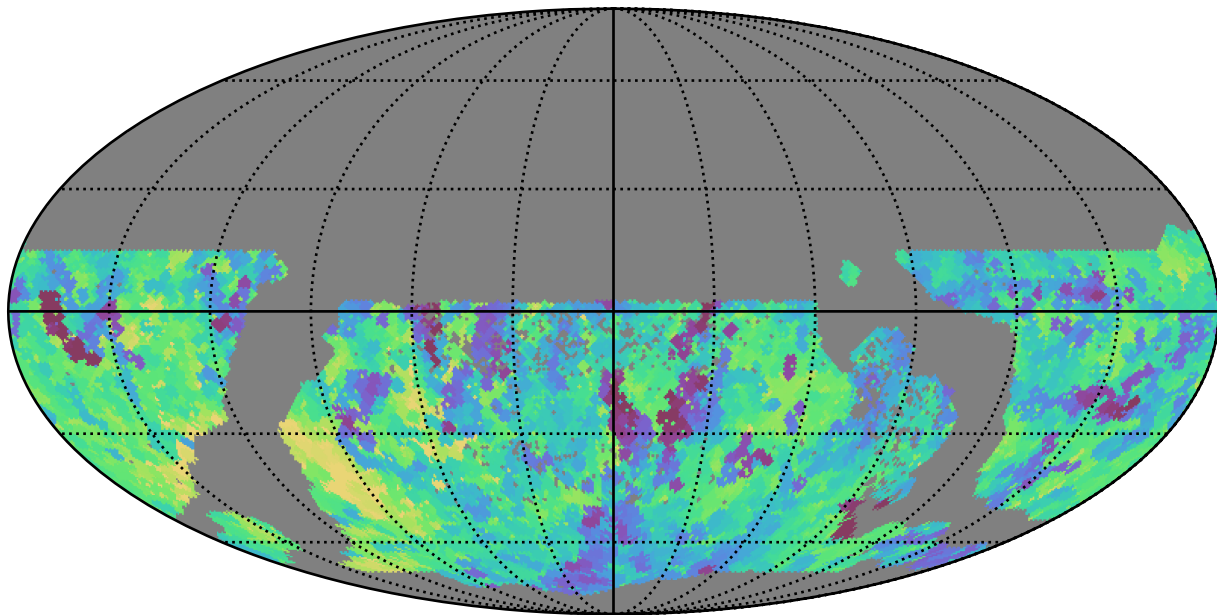
all_long_v3.4_10yrs WFD i band: Min saturation_mag
